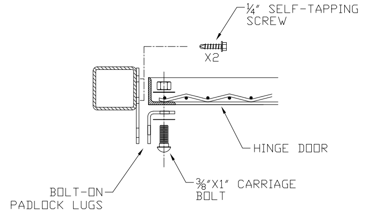
DETAIL OPTIONAL PADLOCK LUGS
